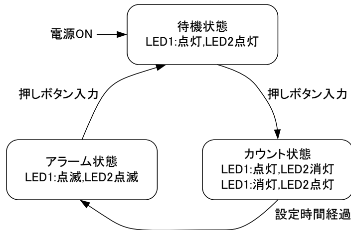
図. 4.2: アラームタイマの状態遷移図
