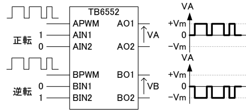
図. 5.5: PWM 信号と出力電圧の関係
