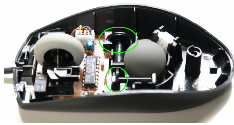
図. 6.3: ボール式マウスの中のロータリエンコーダ
