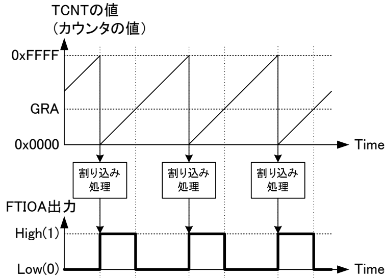
図. 5.8: コンペアマッチと割り込みを併用したパルス生成
