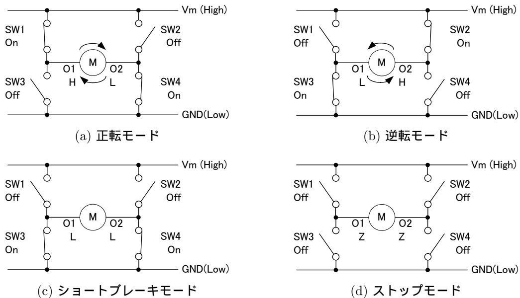
図. 5.3: Hブリッジ回路の基本モード, Zはハイインピーダンスを表す
