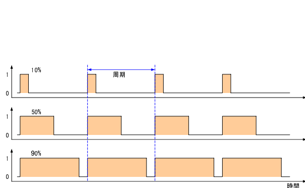
図. 5.1: PWMの例
