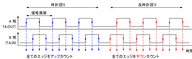
図. 6.5: ロータリエンコーダの A 相/B 相出力と回転方向識別
