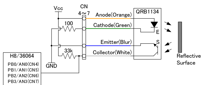
図. 6.1: 赤外線センサとその接続
