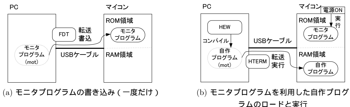
図. 1.1: モニタプログラムを利用し, 自作プログラムを RAM 領域にロード, 実行
