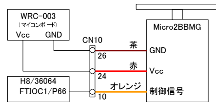
図. 5.7: マイコンボードと RC サーボの接続
