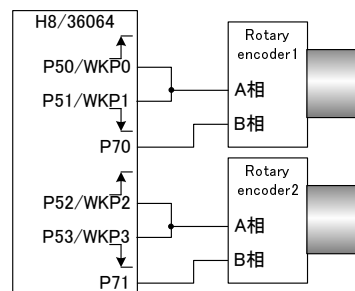
図. 6.7: ロータリエンコーダ 2 つを 2 通倍カウントする場合の接続例
