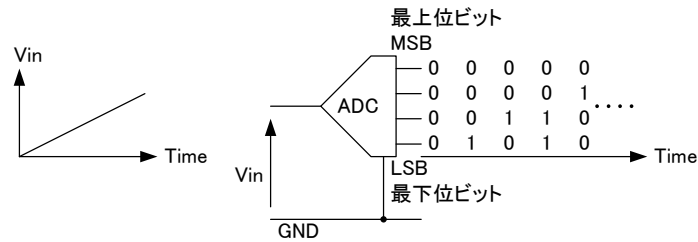
図. 6.2: A/D 変換器の概要
