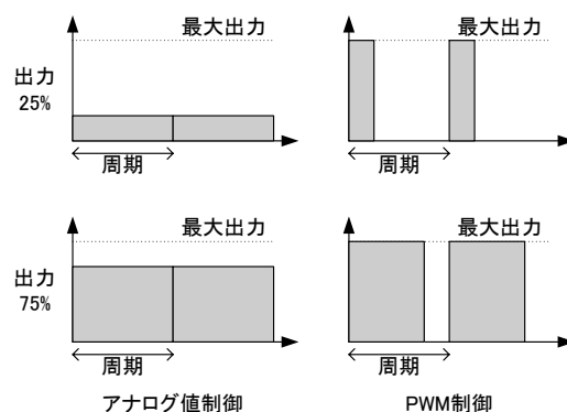
図. 5.2: アナログ値制御とPWM制御の関係
