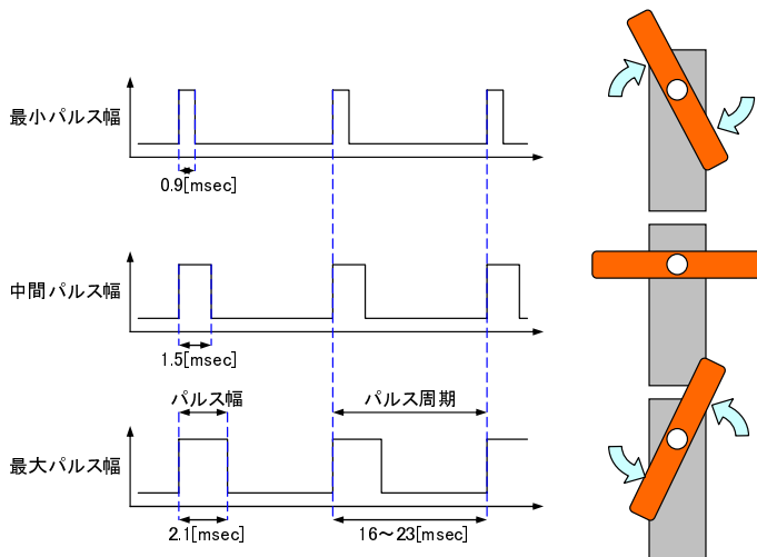
図. 5.6: 制御信号と RC サーボの回転角
