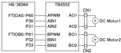
図. 5.4: マイコンとドライバ, モータの接続関係
