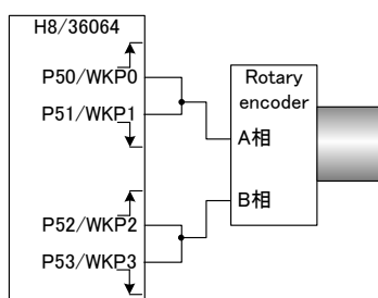
図. 6.6: ロータリエンコーダ 1 つを 4 通倍カウントする場合の接続例
